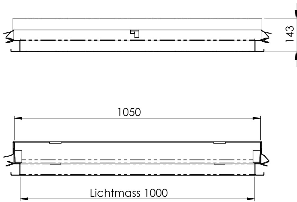
SCHNITT B-B
