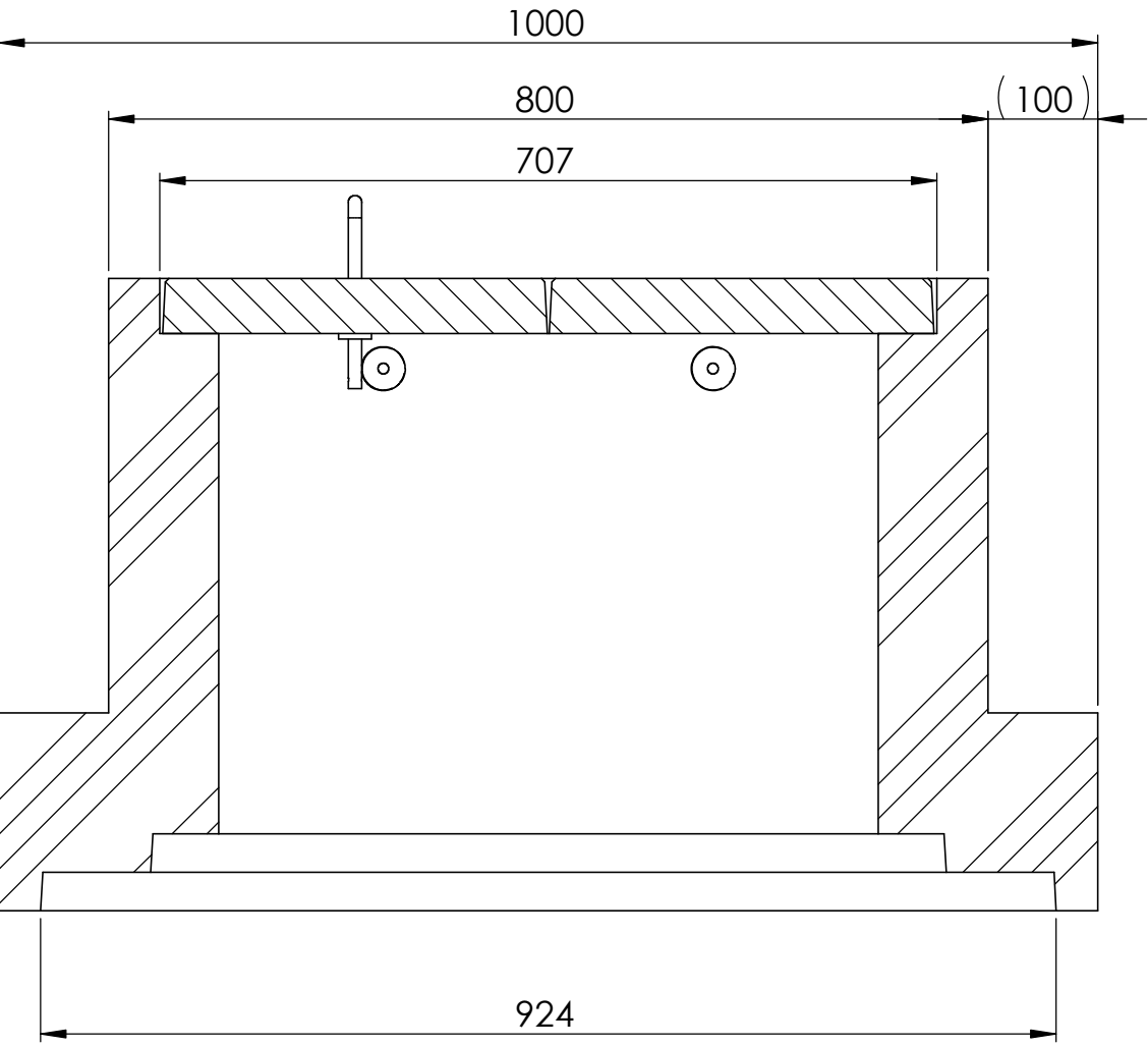
SCHNITT B-B MAßSTAB 1 : 7
