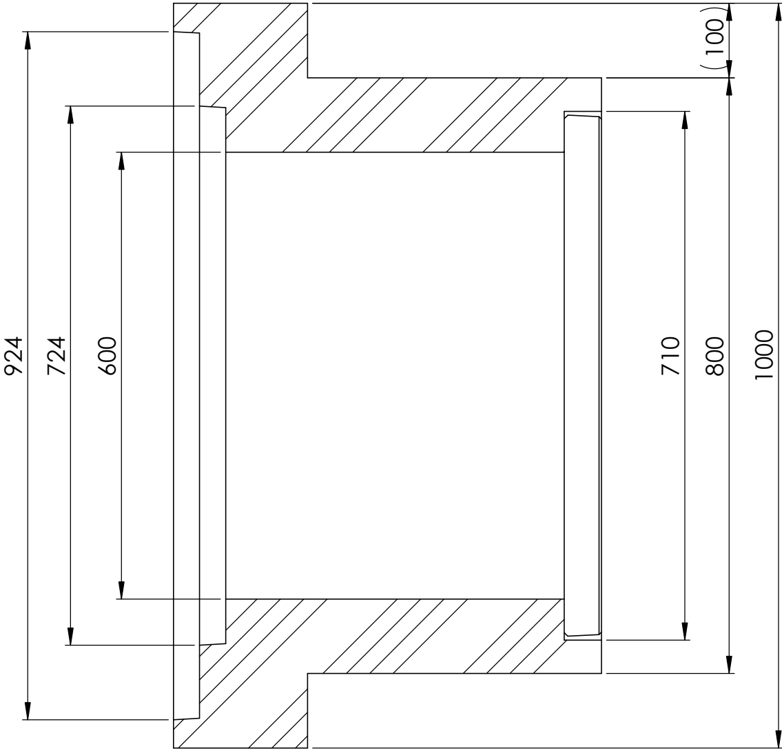
SCHNITT A-A MAßSTAB 1 : 7
