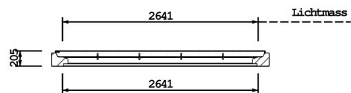
SCHNITT A-A
