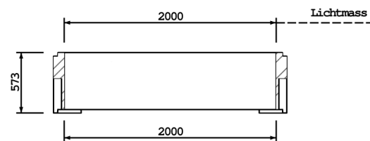
SCHNITT A-A
