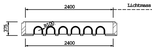
SCHNITT A-A
