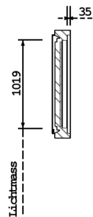
SCHNITT B-B
