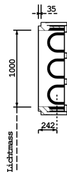
SCHNITT B-B
