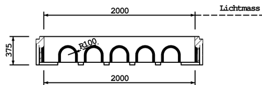
SCHNITT A-A
