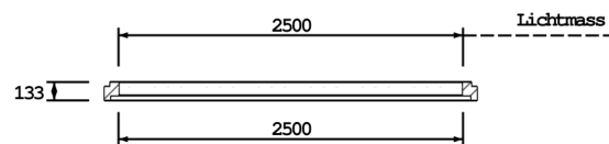
SCHNITT A-A
