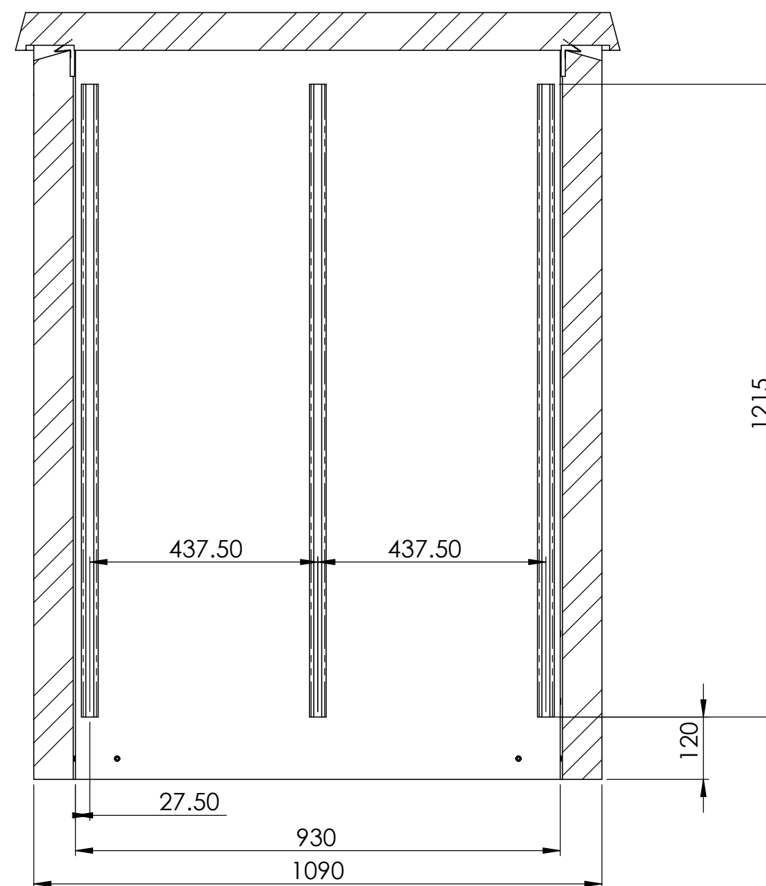
SCHNITT A-A MAßSTAB 1 : 10
