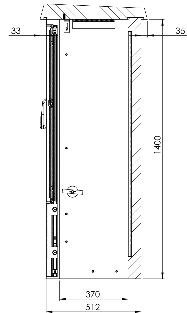
SCHNITT B-B MAßSTAB 1 : 10
