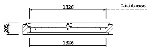
SCHNITT A-A
