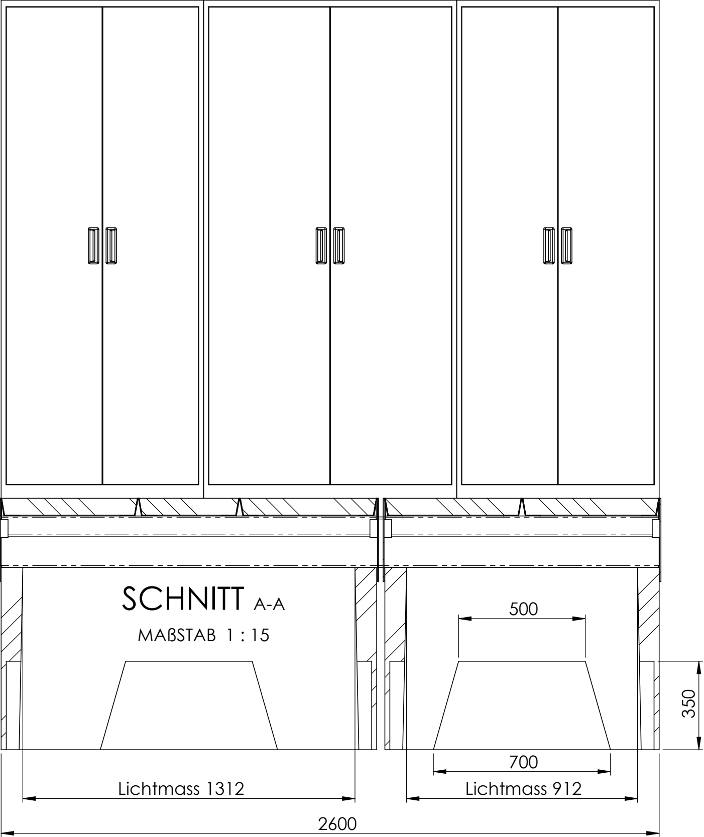
Unterbau für kabine 2600x600x200x4
