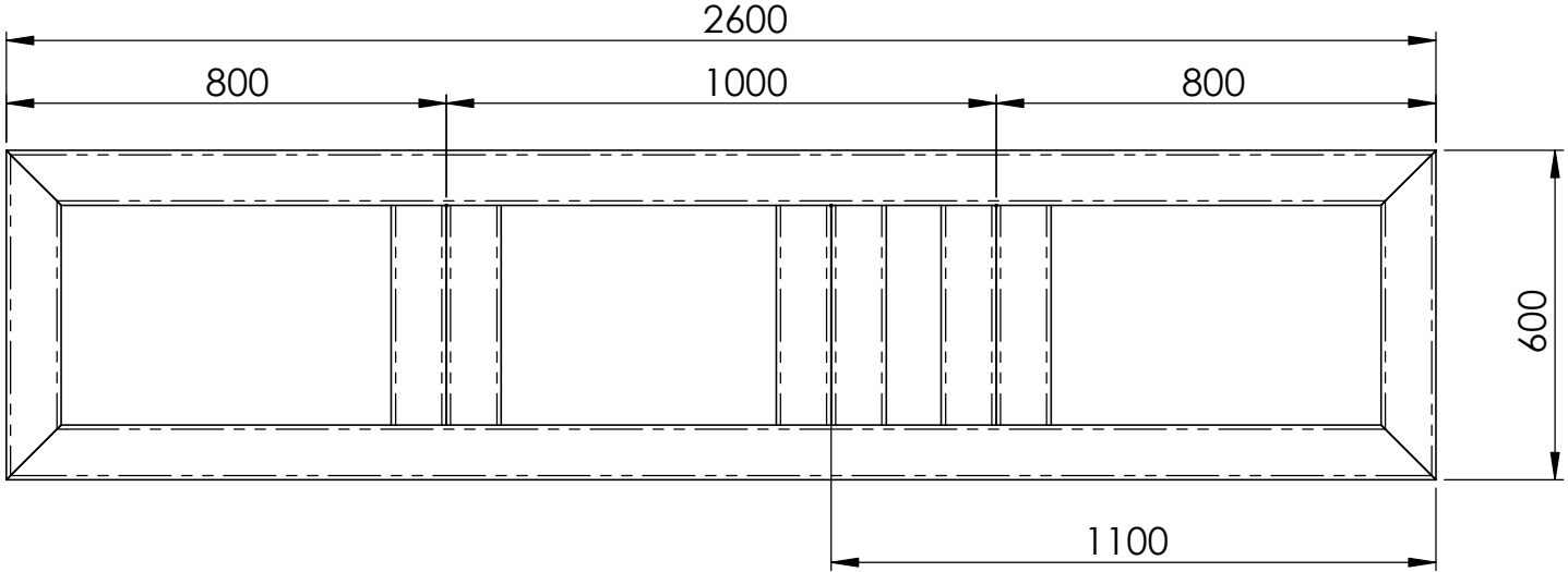
Unterbau für kabine 2600x600x200x4
