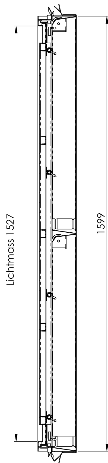
SCHNITT A-A MABSTAB 1 : 8
