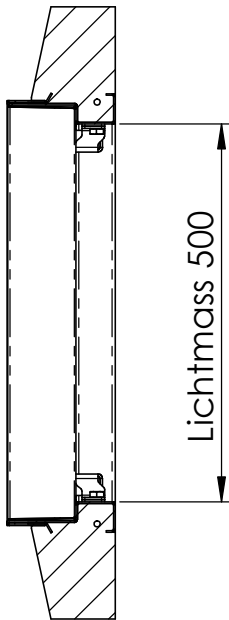
SCHNITT A-A
