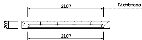
SCHNITT A-A
