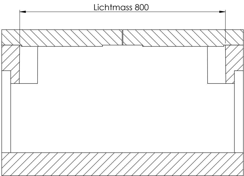
SCHNITT B-B MAßSTAB 1 : 7
