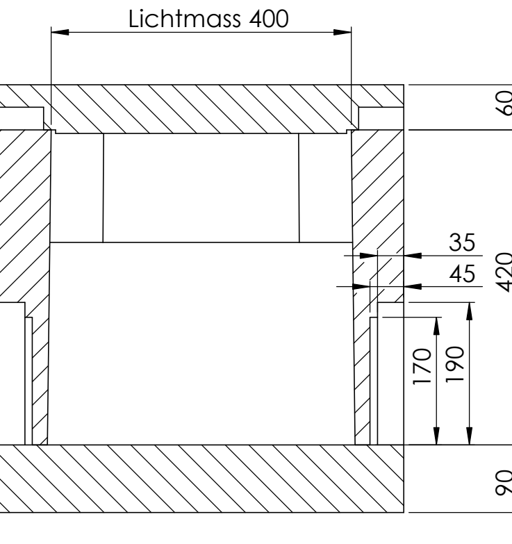
SCHNITT A-A MAßSTAB 1 : 7
