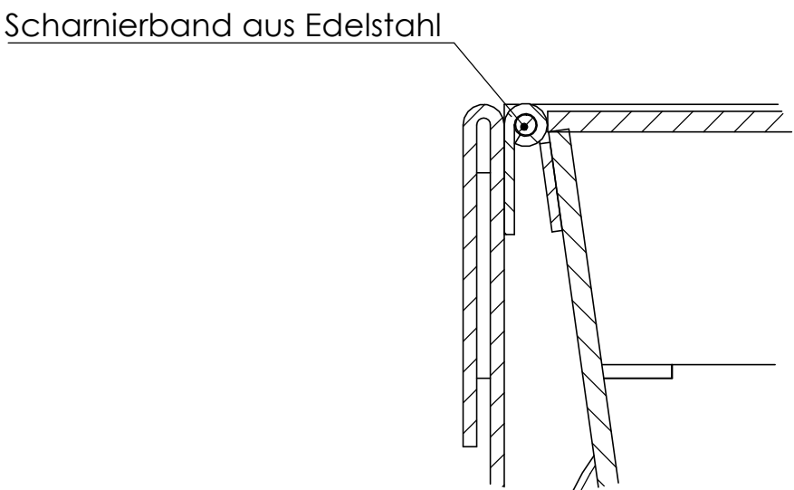
DETAIL C MAßSTAB 1 : 1
