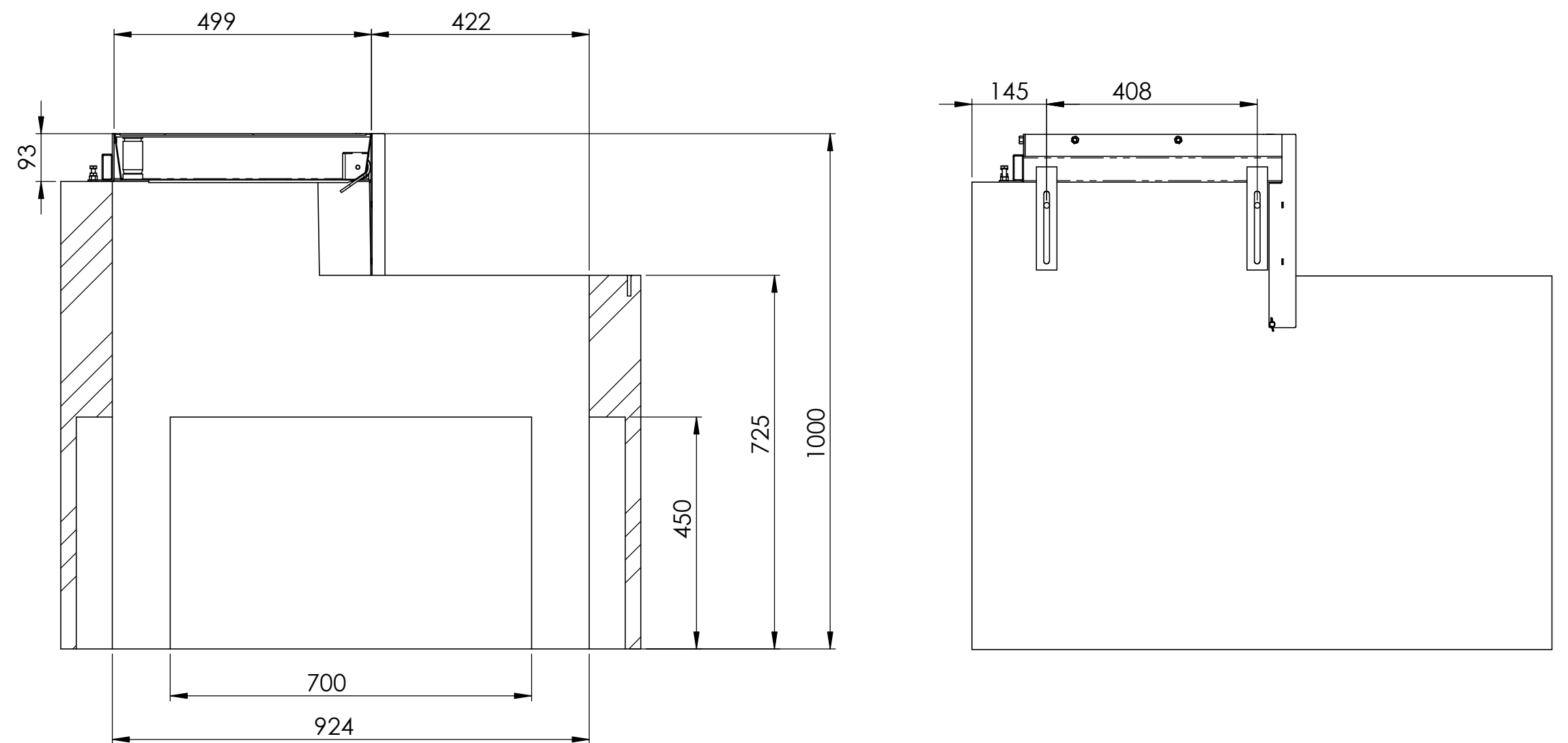
SCHNITT A-A
