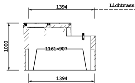
SCHNITT A-A
