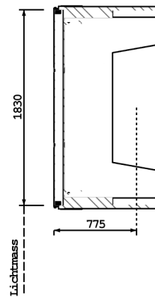
SCHNITT B-B
