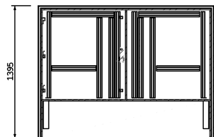
SCHNITT A-A
