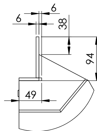
DETAIL C MABSTAB 1 : 5
