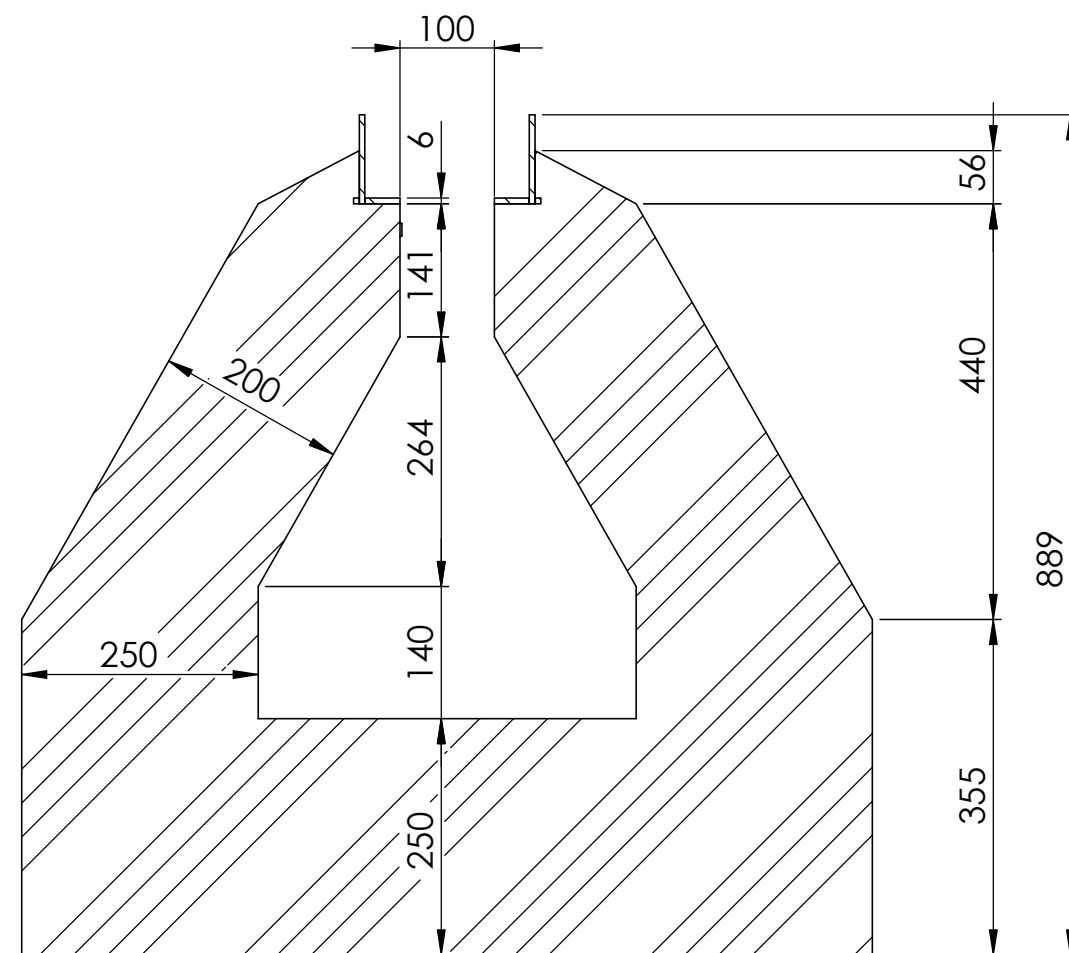
SCHNITT B-B MABSTAB 1 : 8
