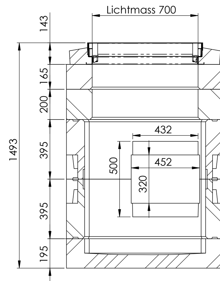
SCHNITT B-B MAßSTAB 1 : 15
