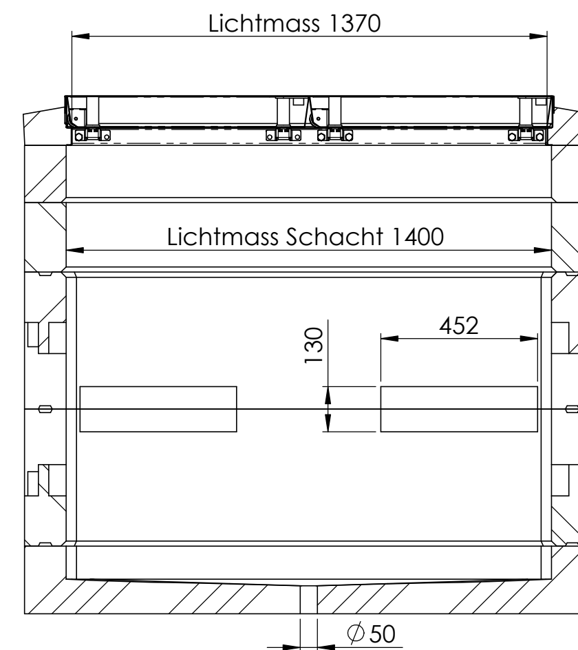
SCHNITT A-A MAßSTAB 1 : 15
