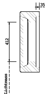
SCHNITT B-B
