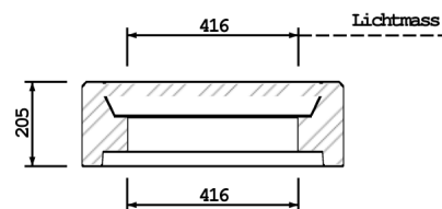
SCHNITT A-A
