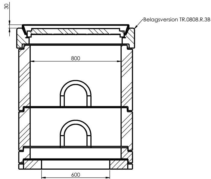
M-M (1 : 10)
