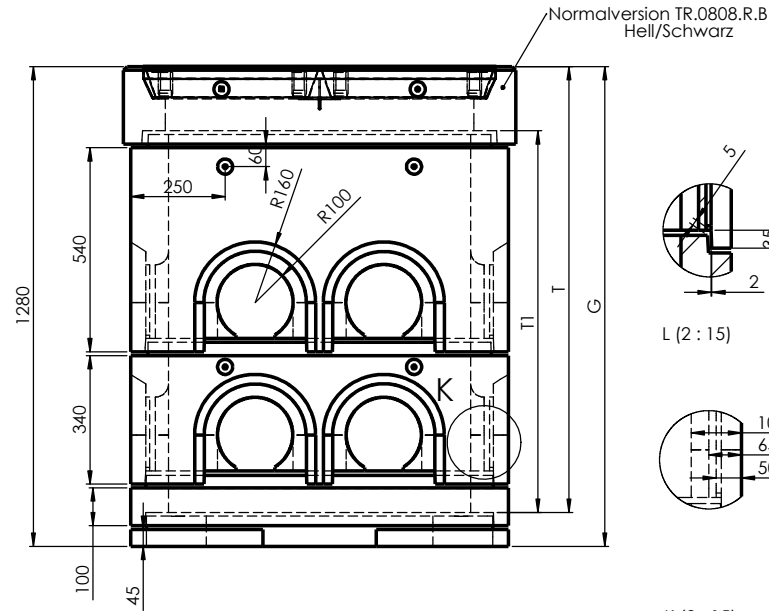
K (2 : 15)
