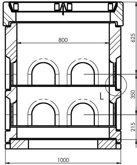
F-F (1 : 10)
