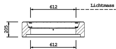
SCHNITT A-A
