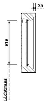
SCHNITT B-B
