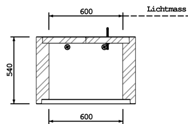
SCHNITT A-A
