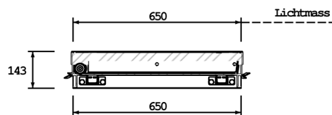
SCHNITT A-A
