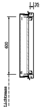
SCHNITT B-B
