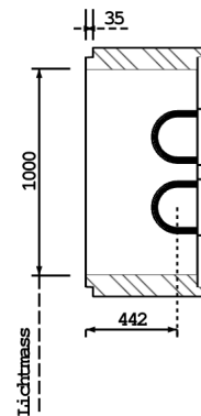
SCHNITT B-B
