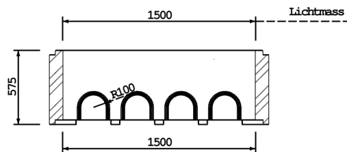
SCHNITT A-A
