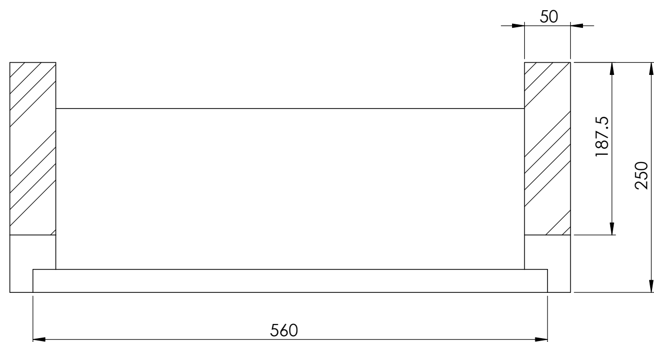
SCHNITT A-A
