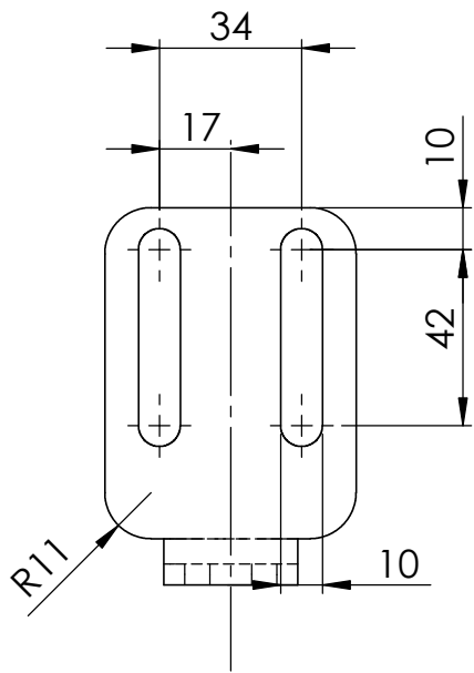
Winkel für C-Leiste-mitte
