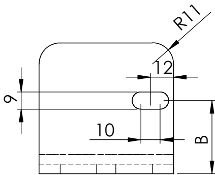
Winkel für C-Leiste-mitte
