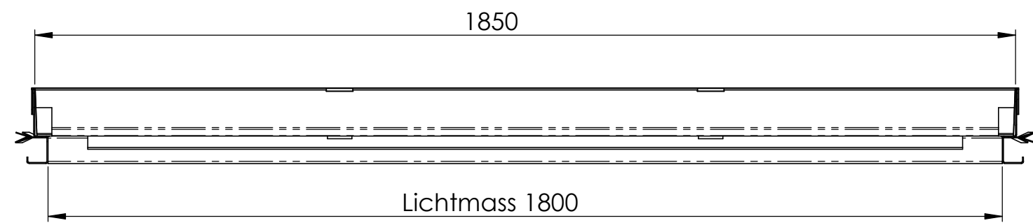
SCHNITT B-B
