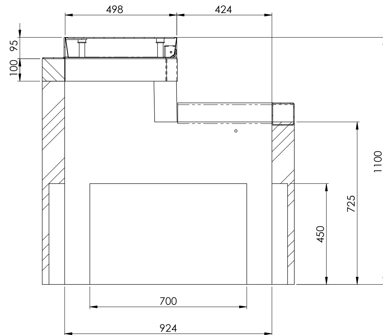
SCHNITT B-B
