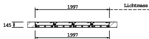
SCHNITT A-A
