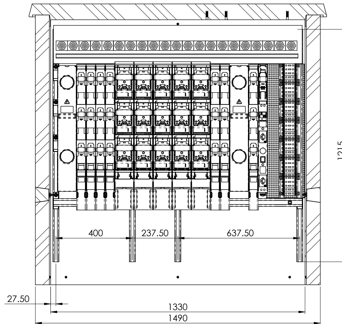
SNITT A-A MABSTAB 1 : 10
