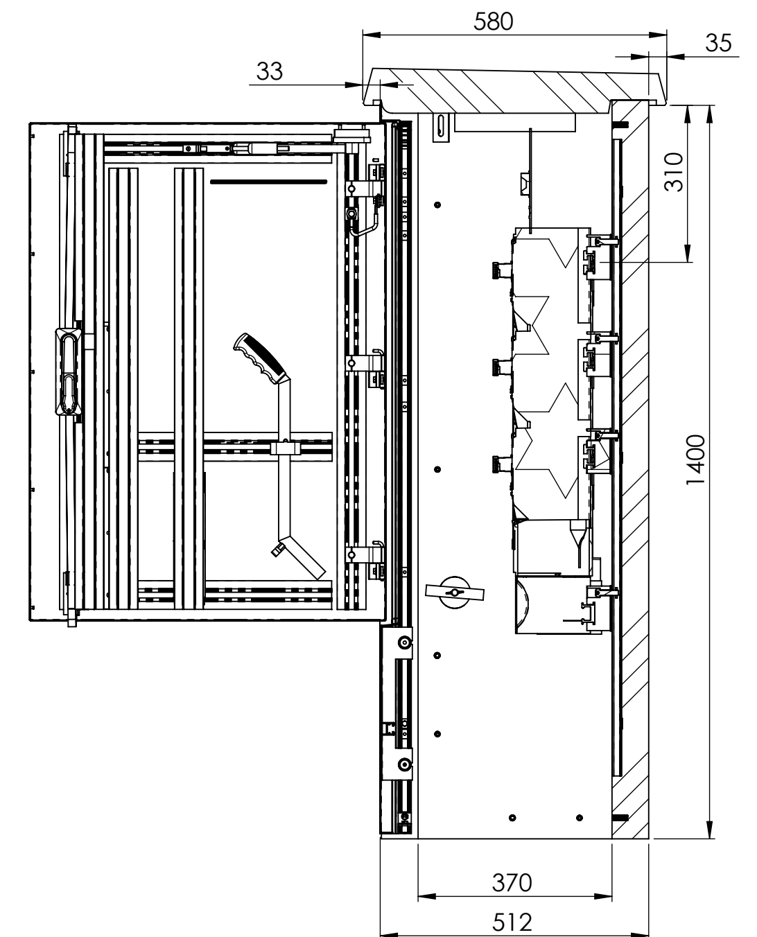
SNITT B-B MABSTAB 1 : 10
