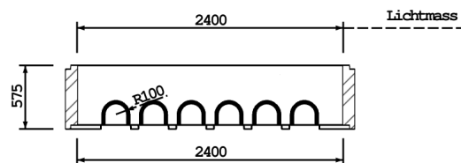
SCHNITT A-A
