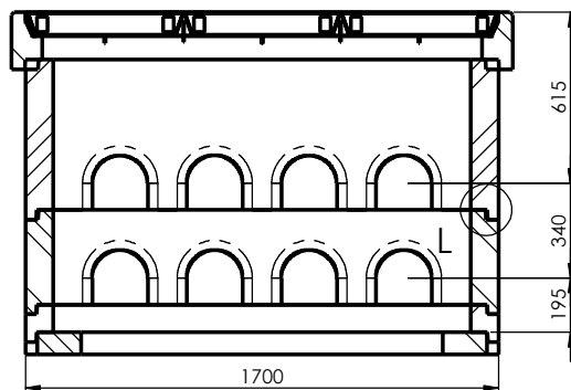
F-F (1 : 15)
