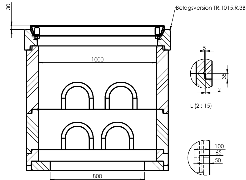
M-M (1 : 10)
