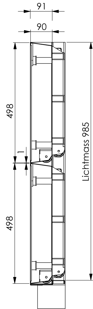
B-B (1 : 8)
