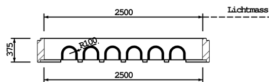
SCHNITT A-A
