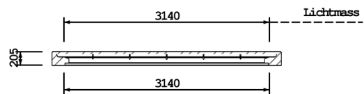
SCHNITT A-A
