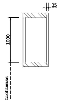
SCHNITT B-B
