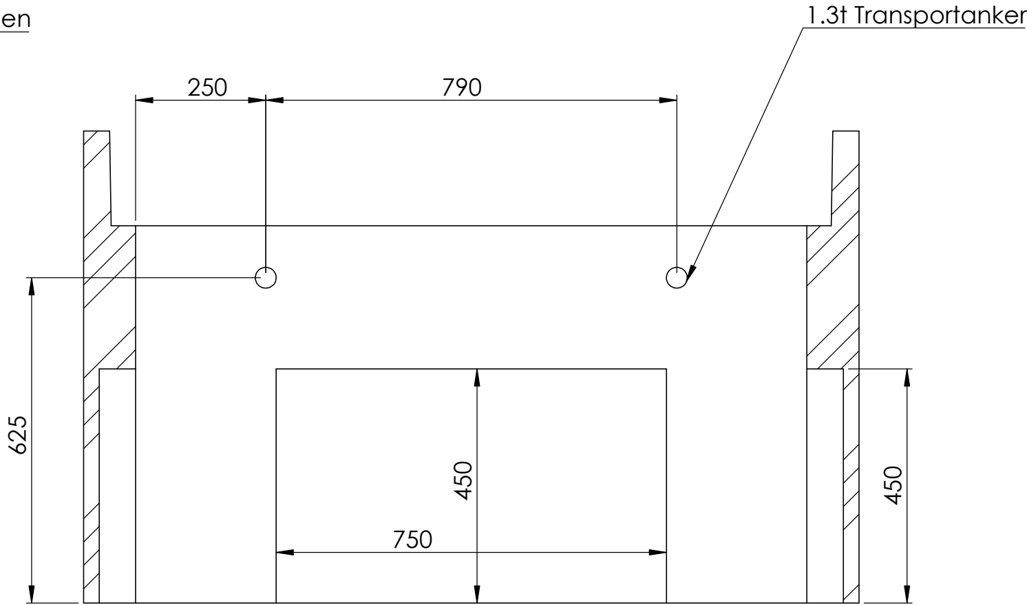
SCHNITT B-B
