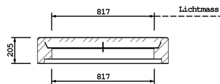
SCHNITT A-A
