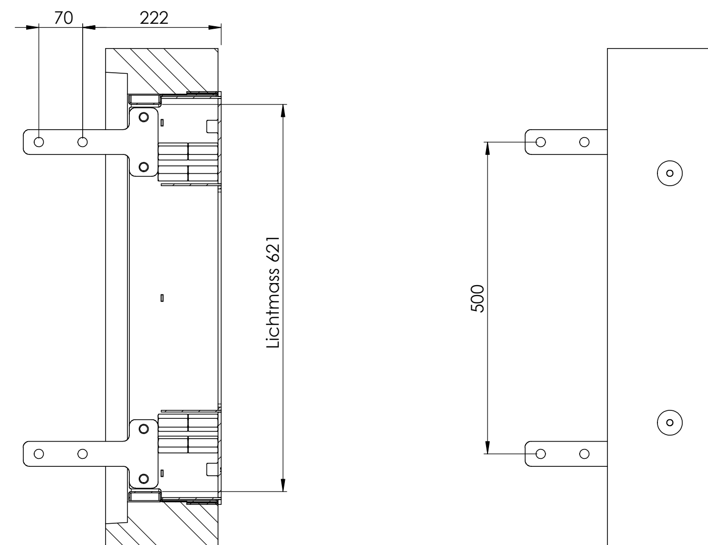
SCHNITT A-A
