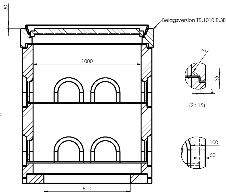
M-M (1 : 10)
