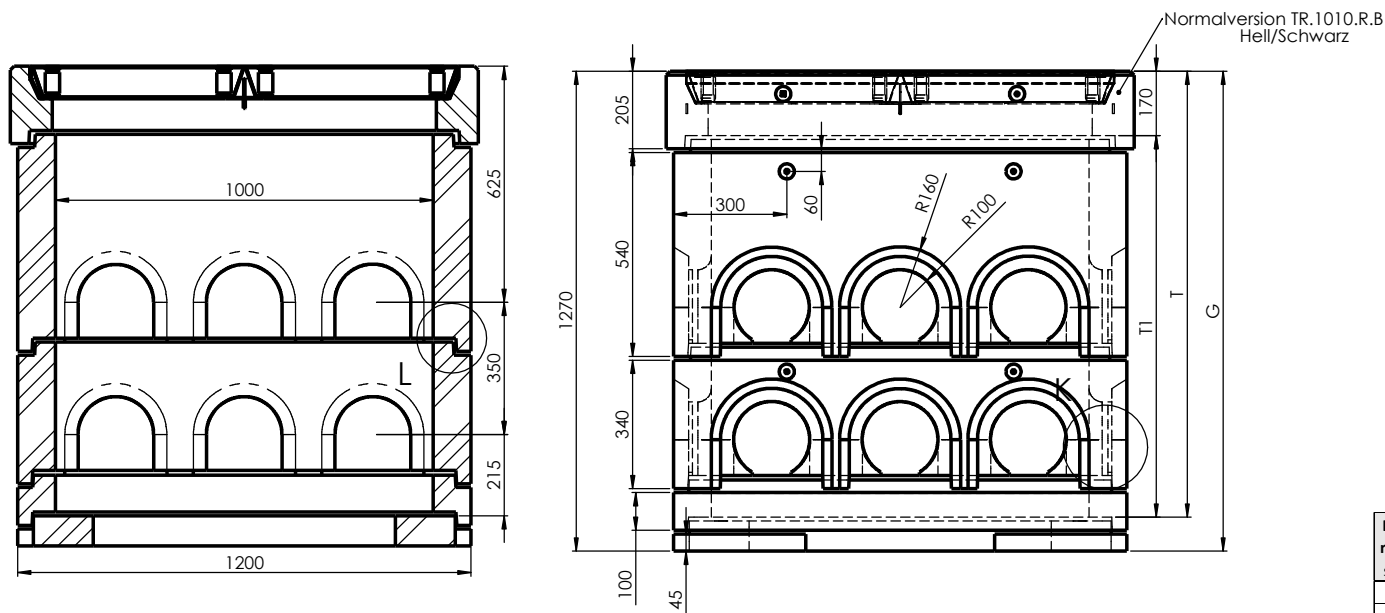
F-F (1 : 10)
