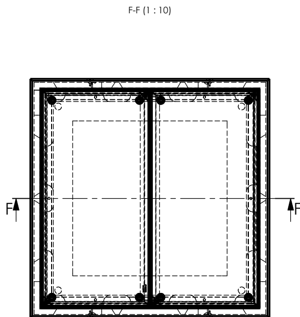
F-F (1 : 10)
