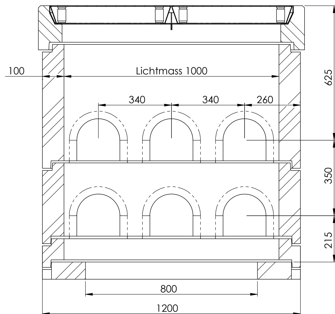
SCHNITT B-B
