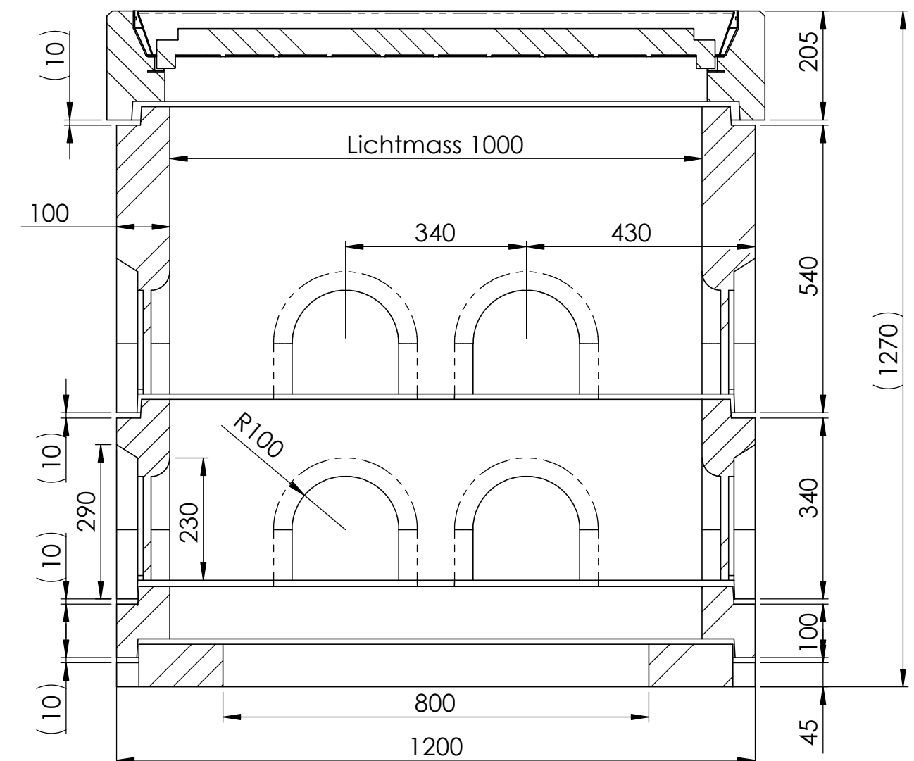
SCHNITT A-A
