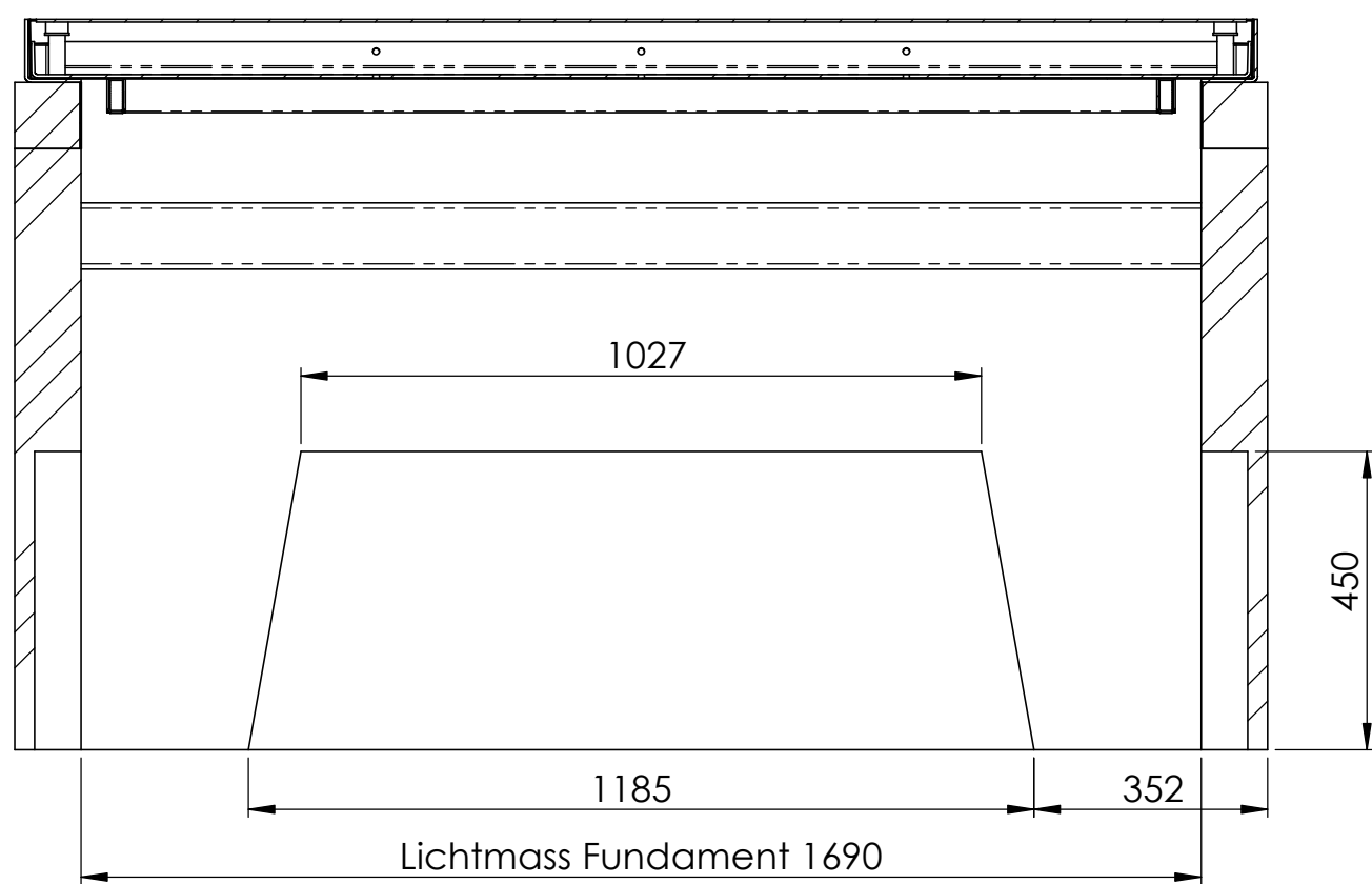
SCHNITT B-B MAßSTAB 1 : 12
