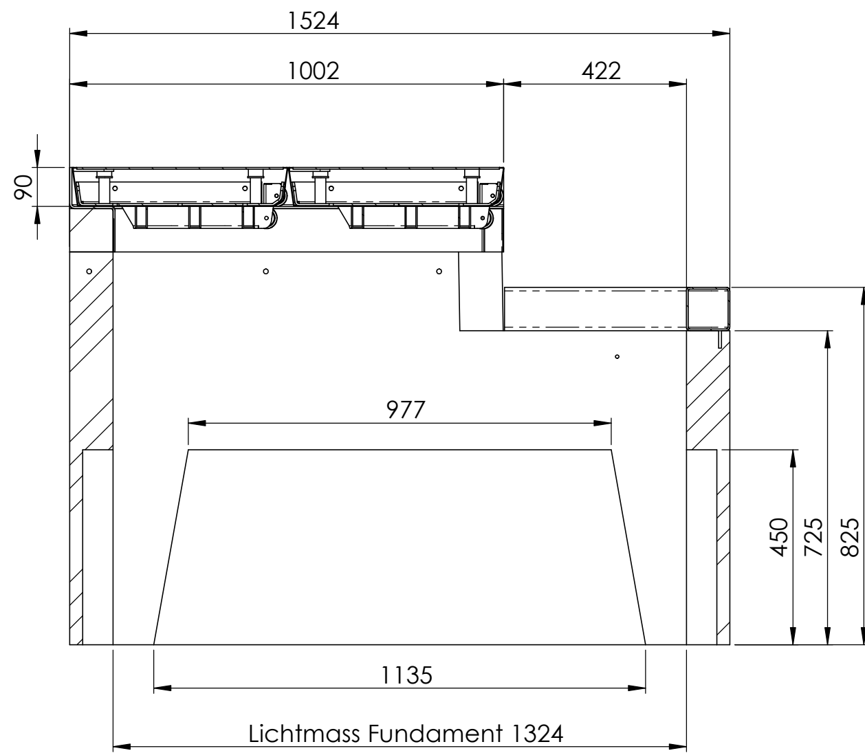
SCHNITT A-A MAßSTAB 1 : 12
