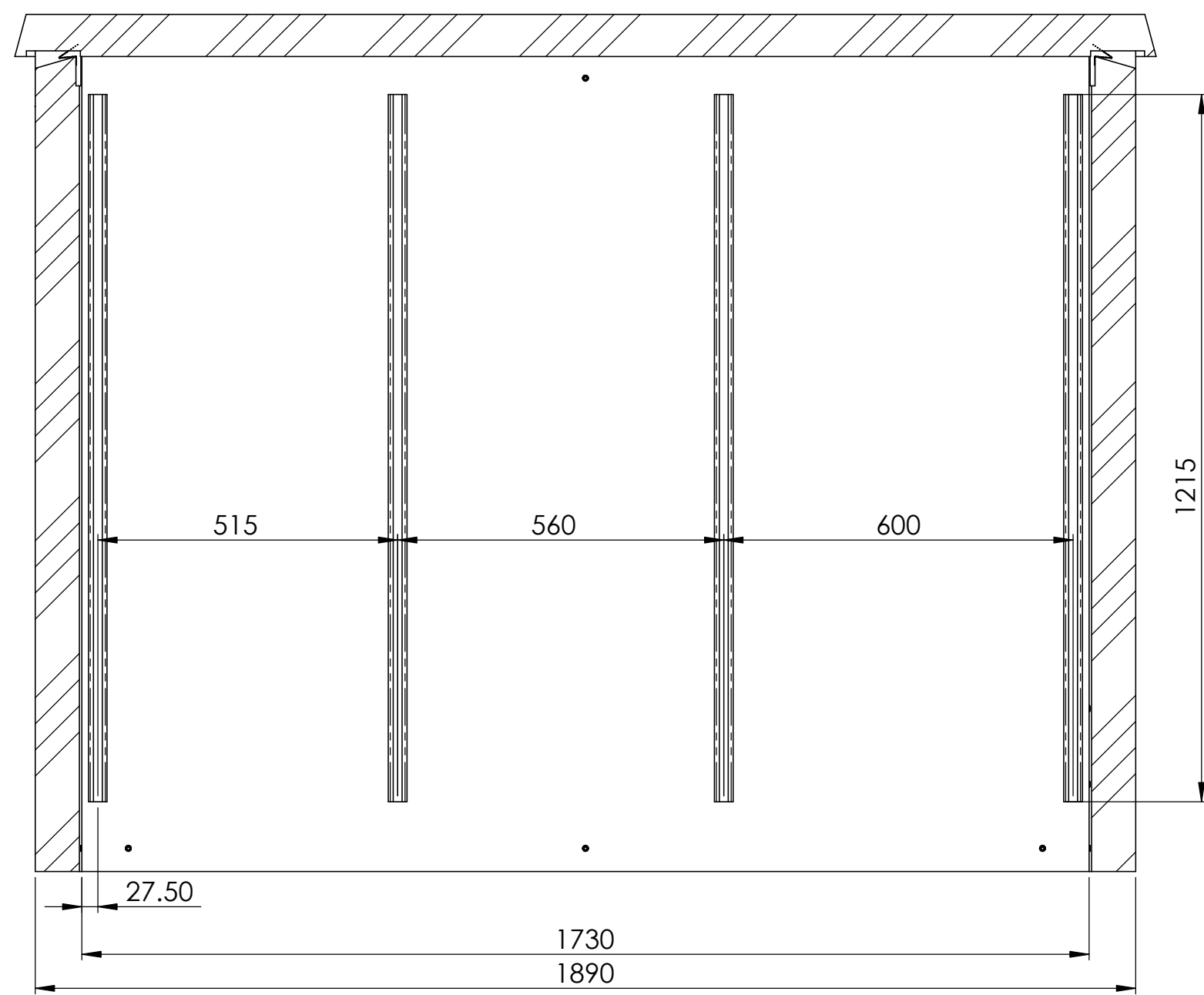
SCHNITT A-A MAßSTAB 1 : 10
