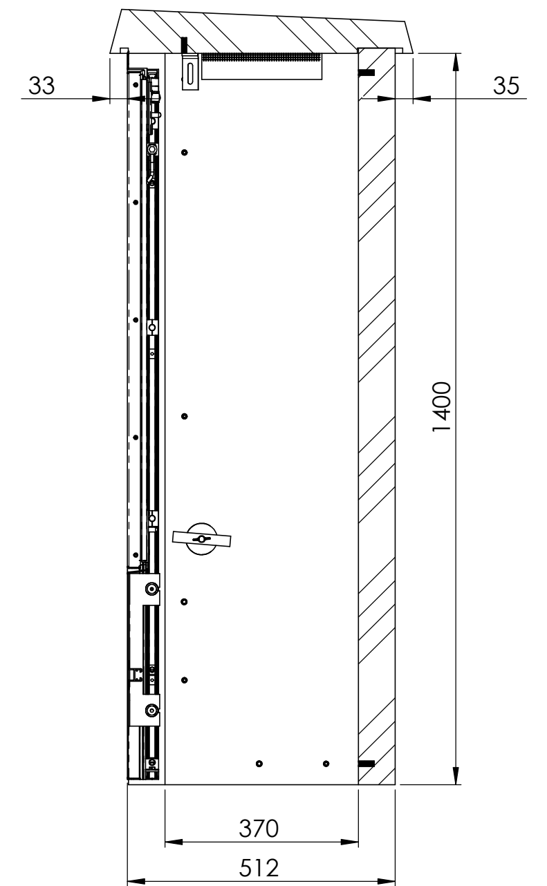
SCHNITT B-B MAßSTAB 1 : 10
