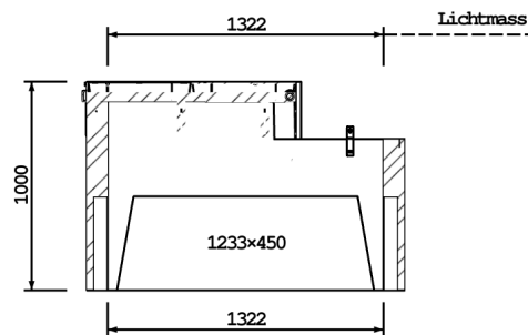
SCHNITT A-A
