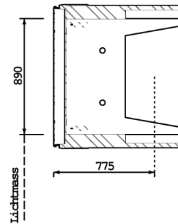
SCHNITT B-B
