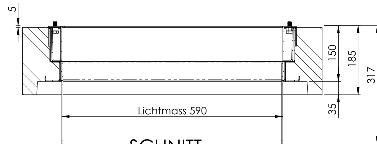
SCHNITT B-B
