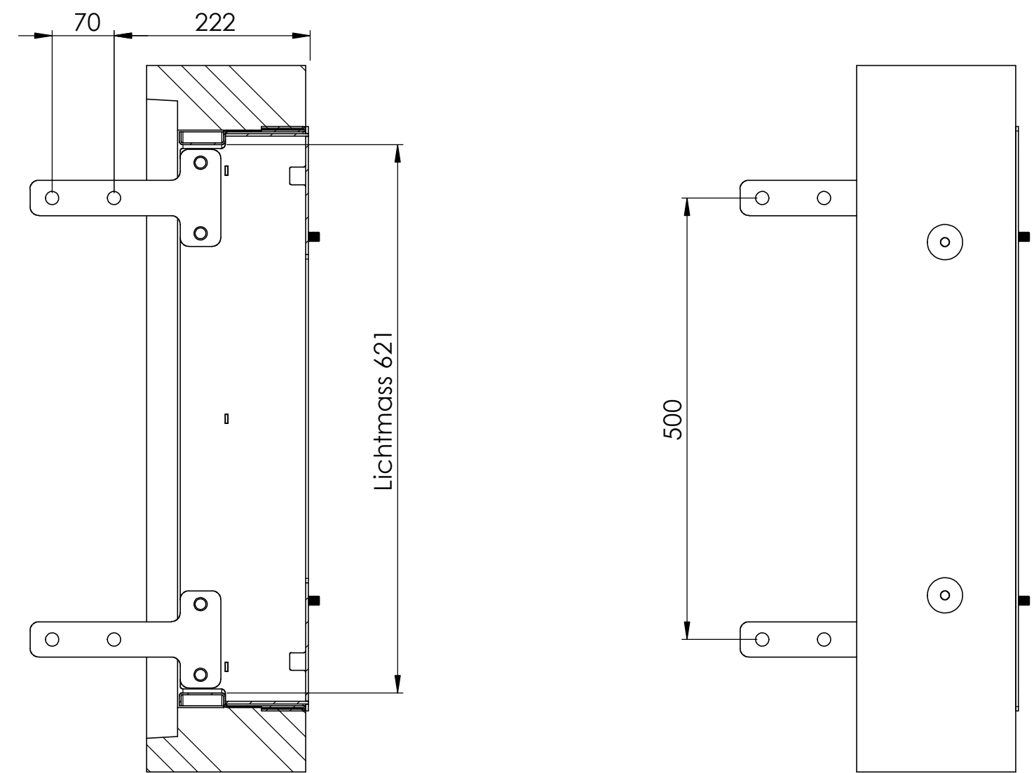
SCHNITT A-A
