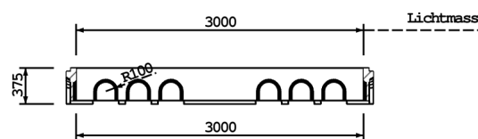
SCHNITT A-A
