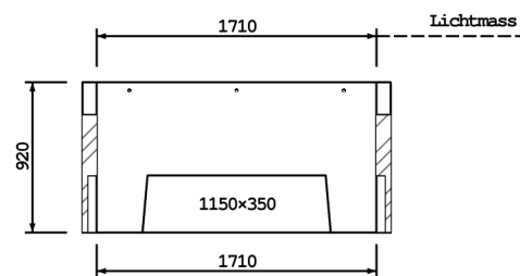
SCHNITT A-A
