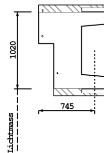
SCHNITT B-B
